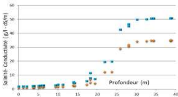
Figure 6 : Profils de salinité (bleu) et conductivité (marron) à travers la lentille d'eau douce (mesures du 22/7/2014 avec une Sonde CDTSE911-couplée d'un ordinateur Vytec-Suunto).
